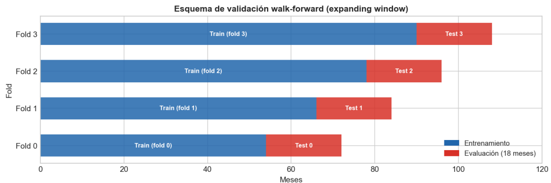
Figura 1. Esquema de validación walk-forward con ventana creciente (expanding window). Cada fila representa un fold; el área azul corresponde al conjunto de entrenamiento y el área roja al horizonte de evaluación de 18 meses.
