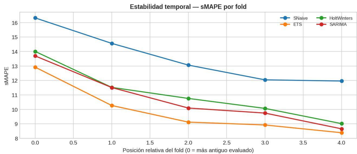
Figura 2. Estabilidad temporal del sMAPE por modelo y fold walk-forward (modelos estadísticos locales).
