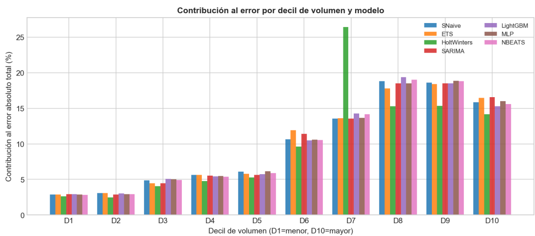
Figura 3. Contribución al error absoluto total por decil de volumen y modelo.
